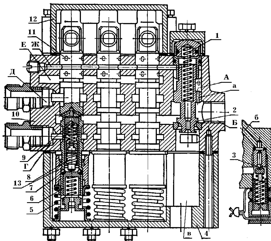
Рисунок 5.3 – Гидравлический распределитель:
