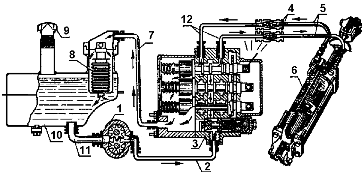
Рисунок 5.1 – Схема простейшей раздельно-агрегатной гидросистемы:
