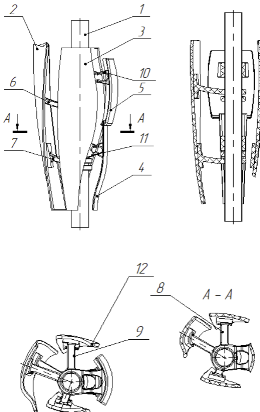
Рисунок 1. Чертёж изделия «SMART-протез»
